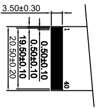
A SC 1:1
